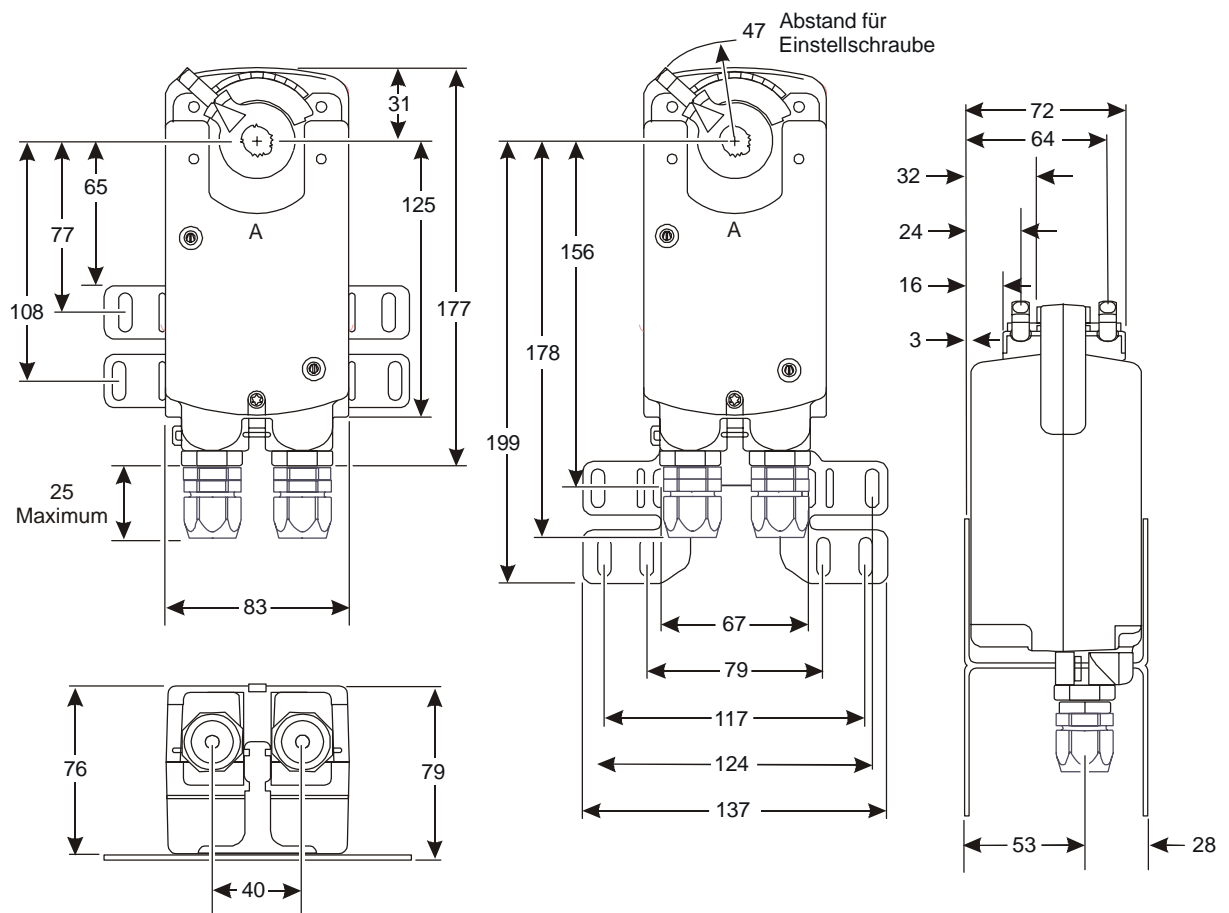
Abbildung 850: Abmessungen (mm) M9206-xxx-1S
